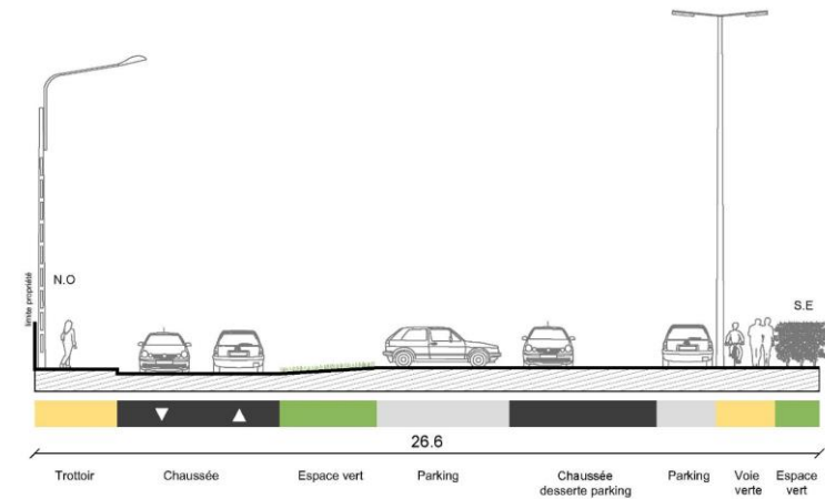
Coupe de l'existant
