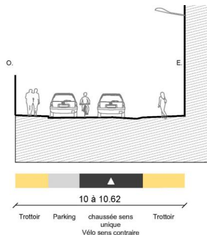
Coupe de l'existant
