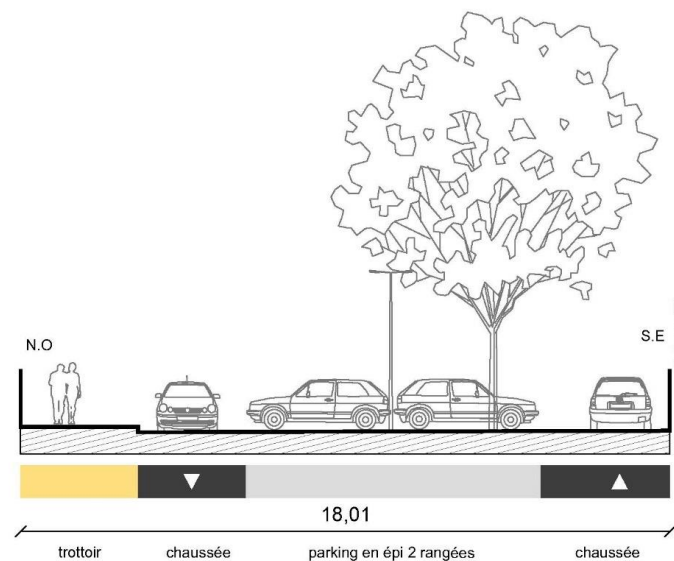
Coupe de l'existant
