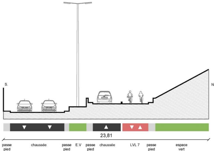
Coupe de la proposition
