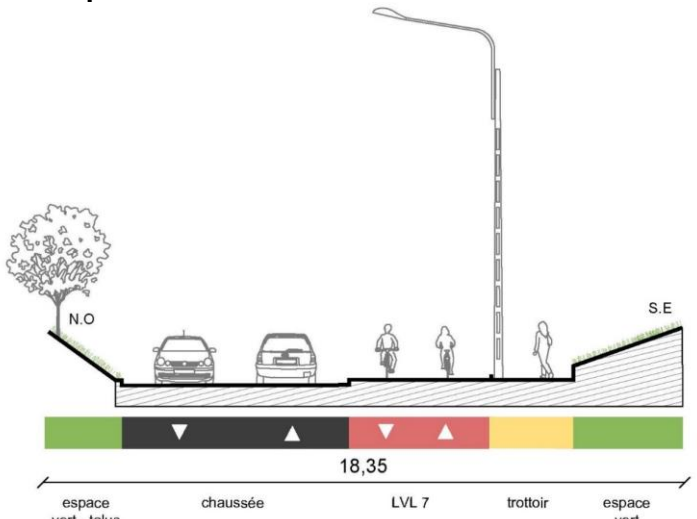
Coupe de la proposition
