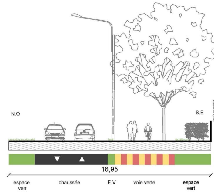
Coupe de la proposition
