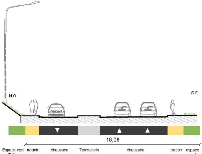
Coupe de l'existant
