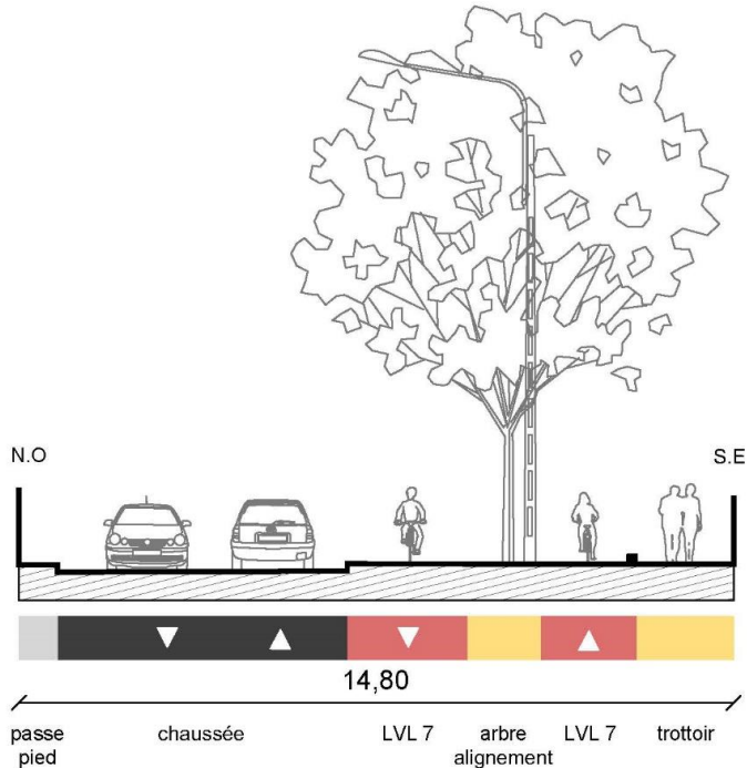
Coupe de la proposition
