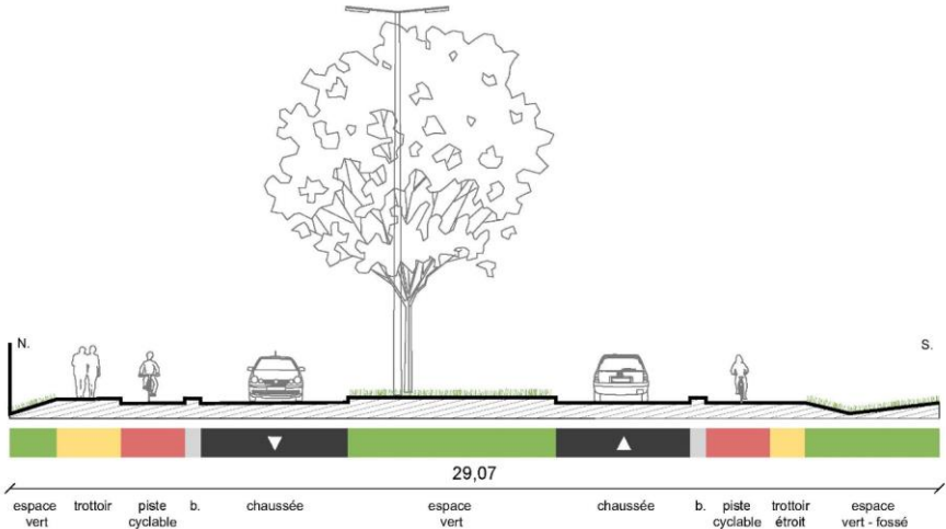
Coupe de l'existant
