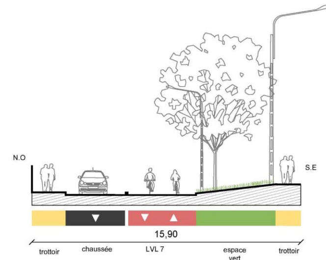
Coupe de la proposition
