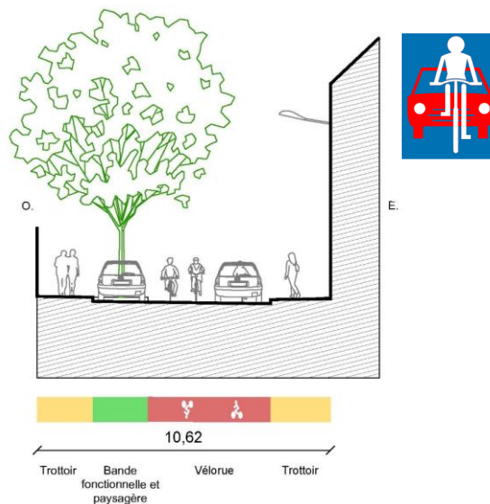
Coupe de la proposition 2
