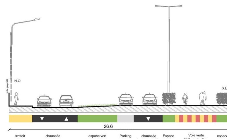
Coupe de la proposition 2
