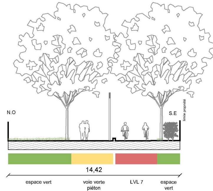
Coupe de la proposition 1
