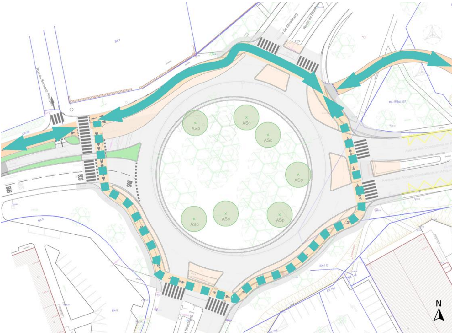
Plan Giratoire Général de Gaulle
