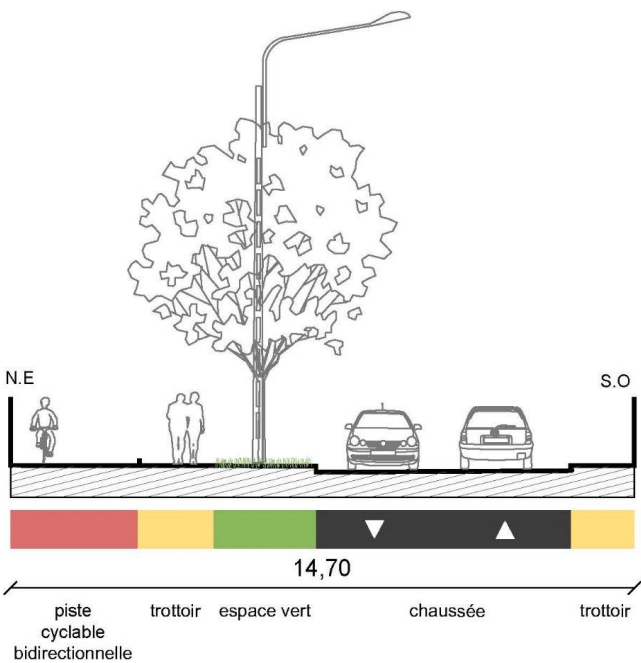
Coupe de l'existant
