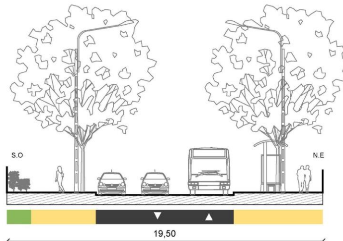
Coupe de l'existant
