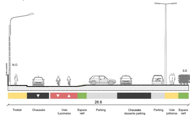
Coupe de la proposition 1
