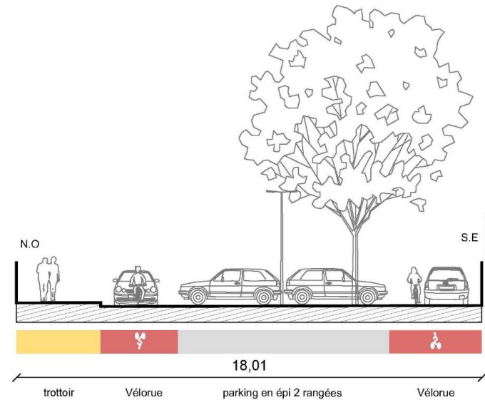
Coupe de la proposition
